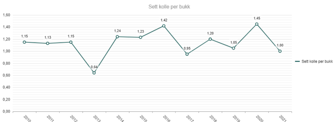
Figur 11: Sett kolle per bukk 2010 - 2021
