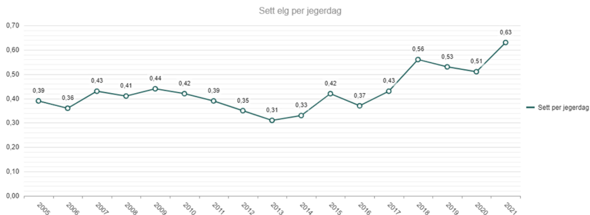
Figur 2: Sett elg per jegerdag 2005 - 2021
