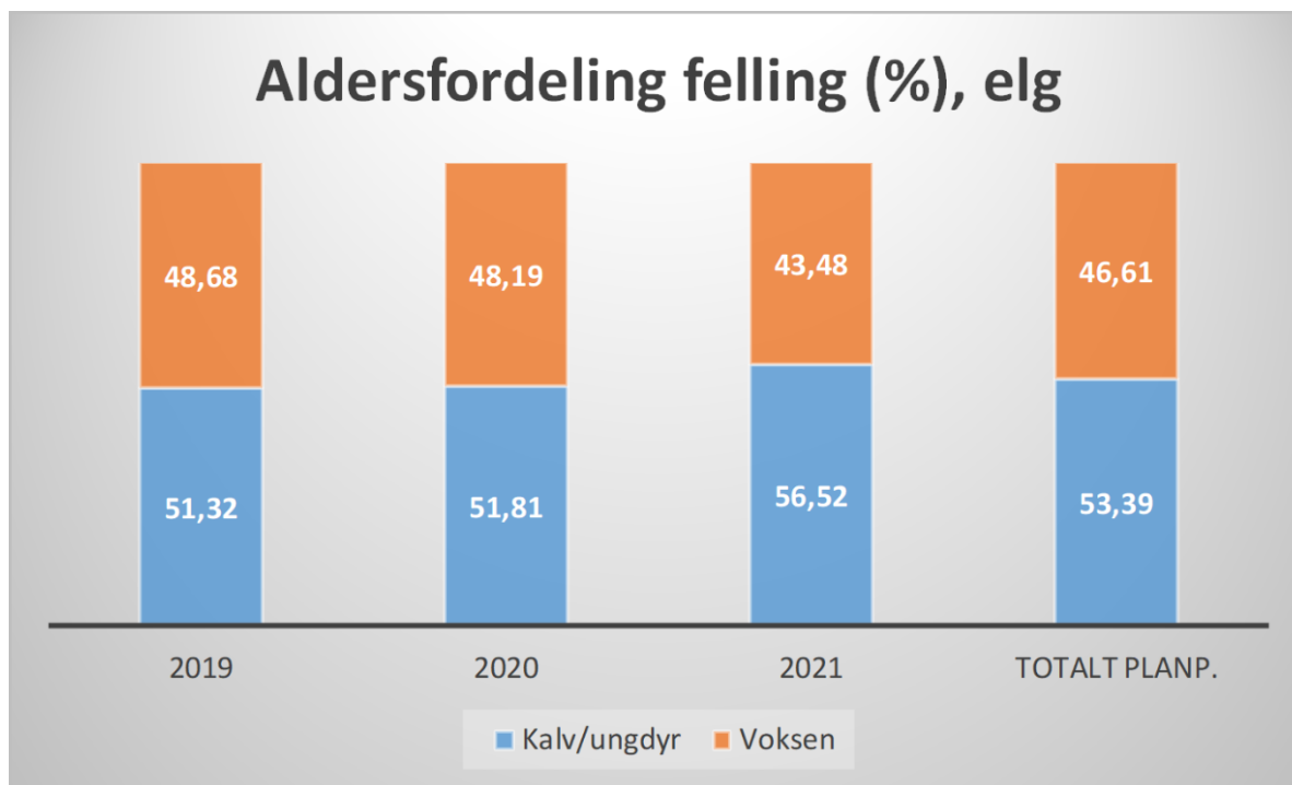
Figur 9: Aldersfordeling på elg i % i planperioden 2019 - 2021
