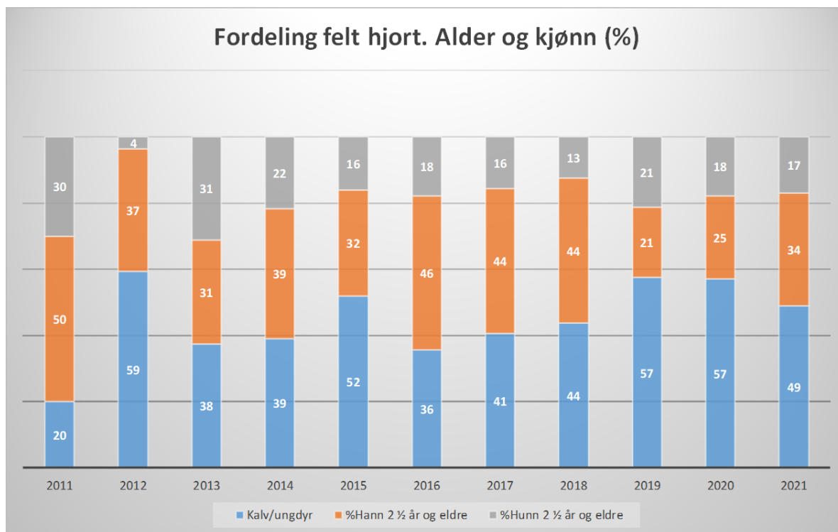
Figur 14: Felt hjort fordelt på alder og kjønn 2011 – 2021 |
