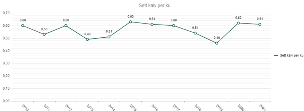
Figur 5: Sett kalv per ku 2010 – 2021
