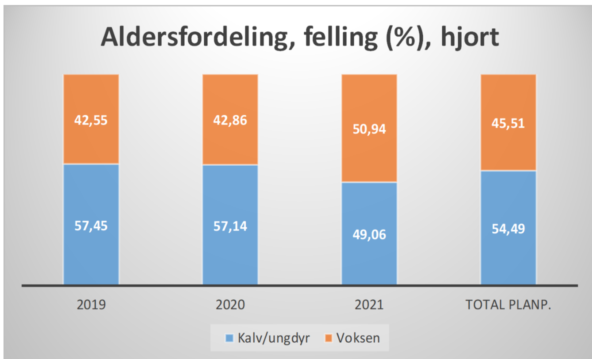
Figur 13: Aldersfordeling i 5 på felt hjort
